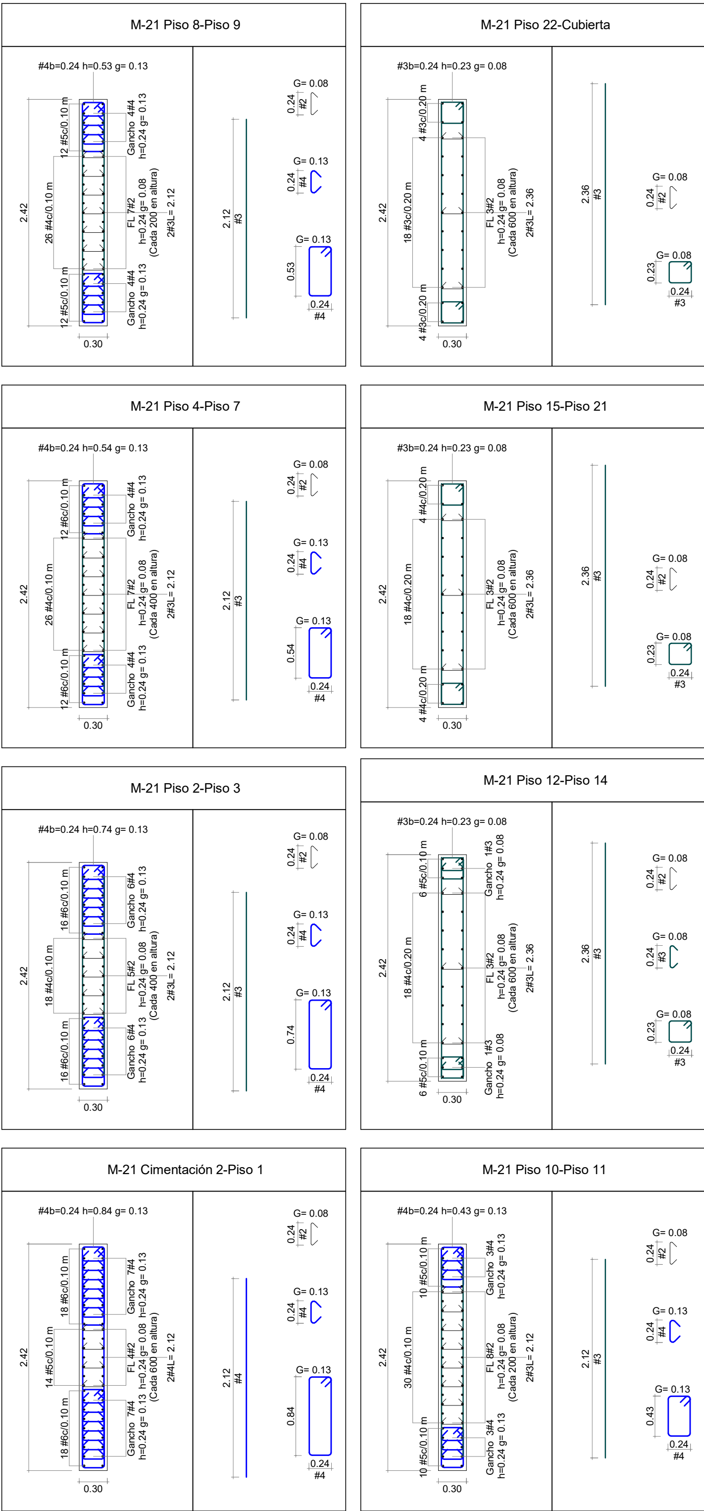
DETALLE SOBRE ANCHO EN MURO M-21 Escala 1 : 25
