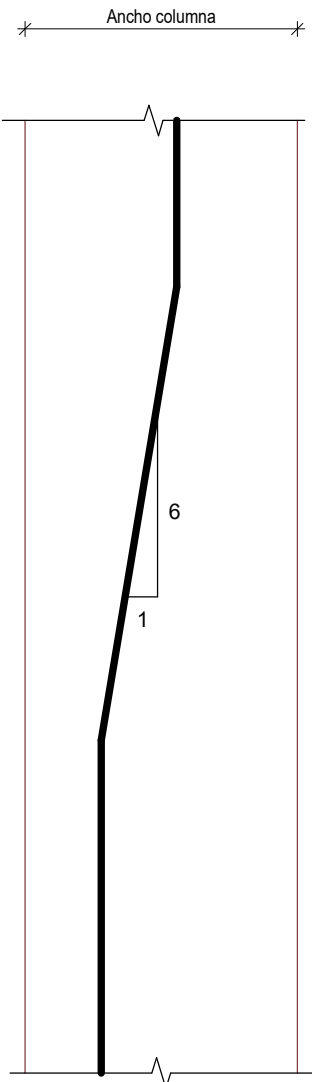
DETALLE DOBLEZ Escala 1 : 10
